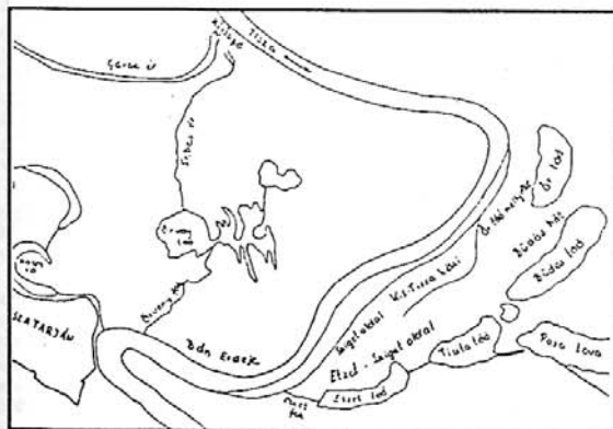
2. ábra Jellegzetes artéri öblözet Tiszatarján határában 3. ábra A Szil-fok öblözete Tiszakeszinél
