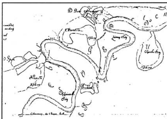
5. ábra Alpár XVIII. századi térképe a fokrendszer nyomaival 6. ábra A Kisvársánytól Tiszadobig terjedő Tisza szakasz XVIII. századi térképének részlete fokokkal és halasokkal
